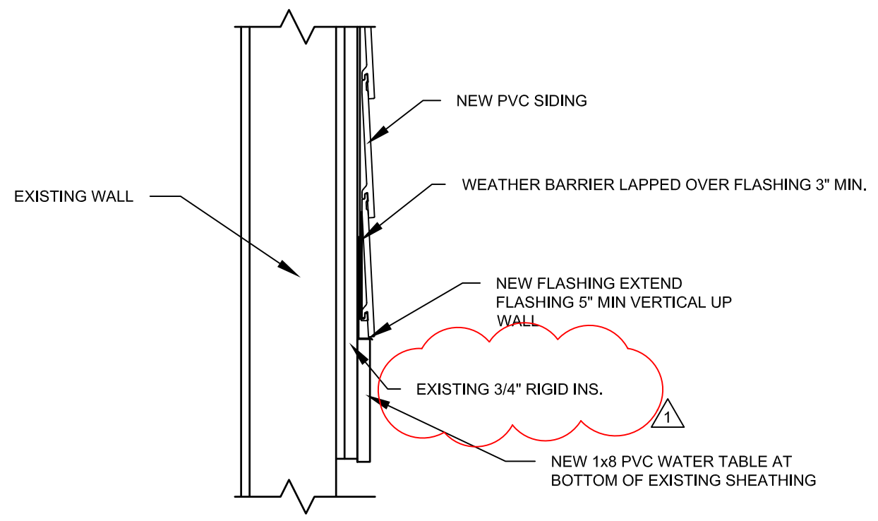
WATER TABLE SCALE: 1 1/2" = 1'-0"
